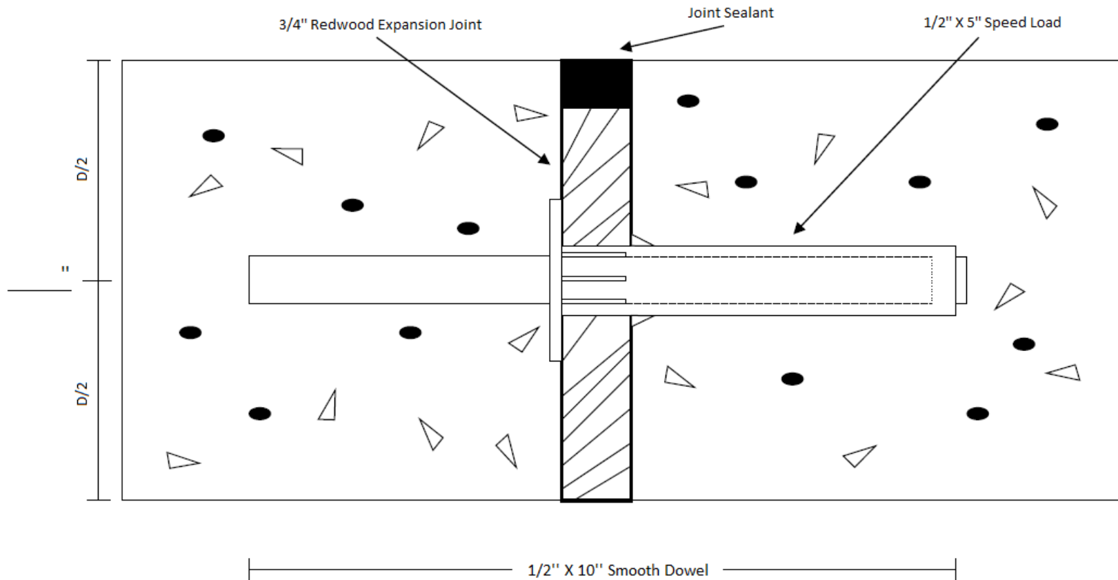
Section View Scale N.T.S
